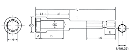
NUT SETTER
